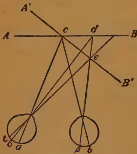
Fig. 17. Binokulare Parallaxe.
